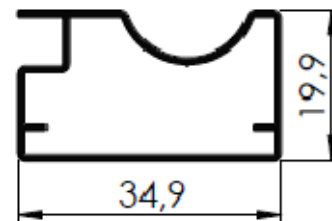
MOLDURA DE ESPELHO
