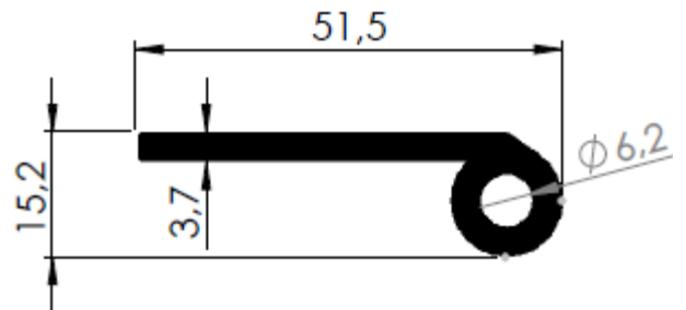
DOBRADIÇA 51,5 x 3,7MM
