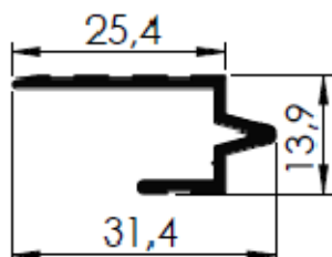
CASE 01 31,4 X 13,9MM
