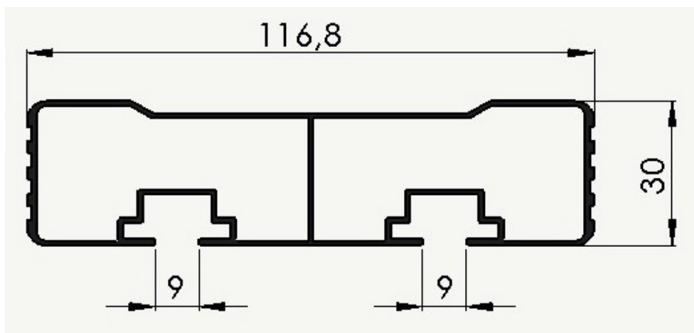
TRAVESSA LATERAL V
