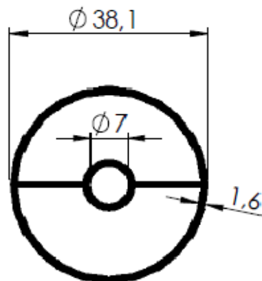
TUBO REDONDO 38,10 COM OLHAL
