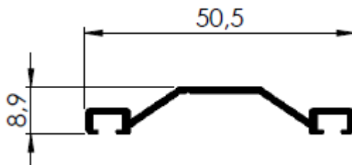
TRAPEZIO PARA POLICARBONATO
