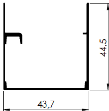
TRILHO SUP. BOX LISO 43,7MMX44,5MM
