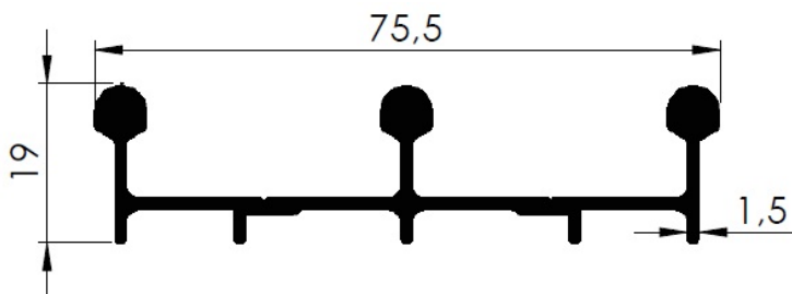
TRILHO TRIPLO P/ CONJUNTO DESLIZANTE
