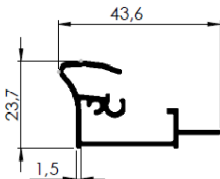
BATE FECHA (BASE 1570)
