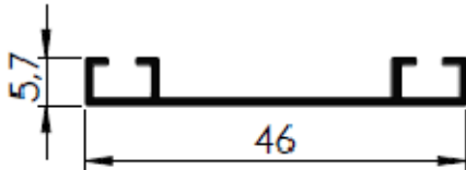
TRILHO INFERIOR 46 X 5,7MMX0,7MM
