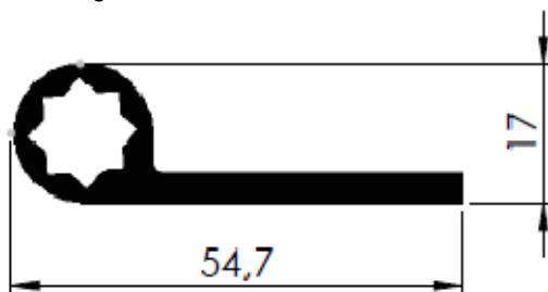
DOBRADIÇA FURO ESTRELA 54,7 X 3,8MM
