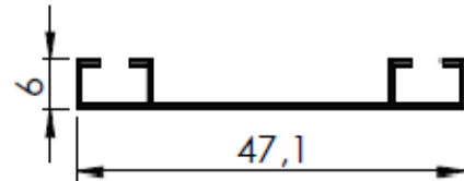
TRILHO INFERIOR 47,1 X 5,7 X 0,7MM
