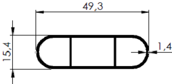
OBLONGO 50 x 15 x 1,4 X 1,4MM
