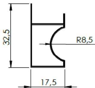
PUXADOR 32,5 X 17,5MM
