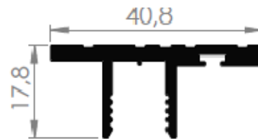
TRANSPASSE 40,8 X 17,8MM
