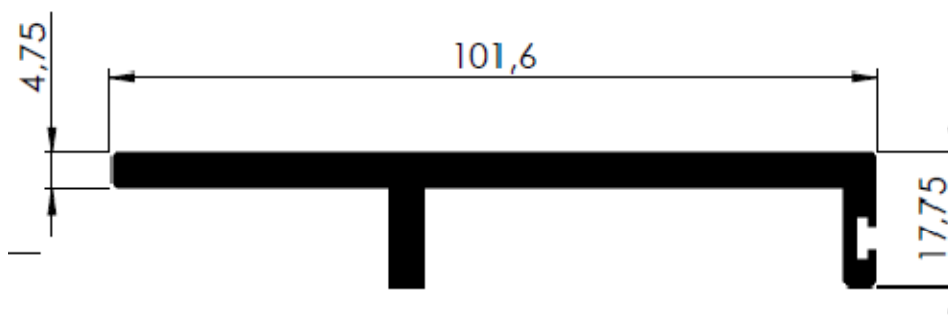
PERFIL "F" DESLIZANTE
