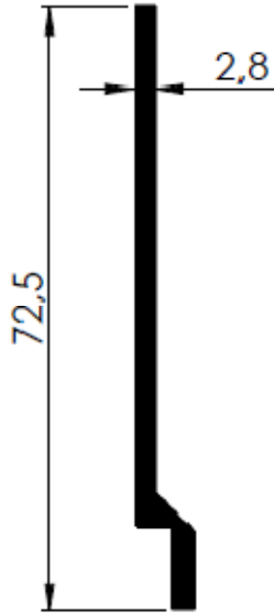
BATENTE 73 x 2,8MM
