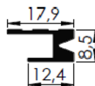
CASE 06 17,9 X 12,4MM
