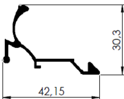
BATE FECHA (FIXO 1570)
