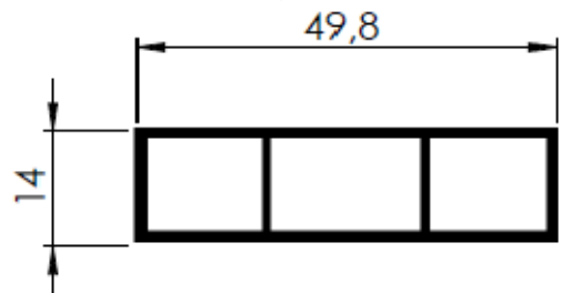
TRAVESSA 49,8 X 14 X 1.2MM
