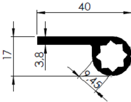
DOBRADIÇA FURO ESTRELA 40 X 3,8MM
