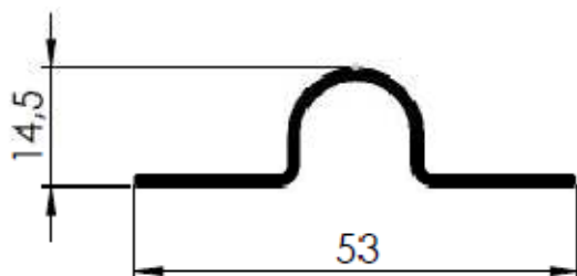
CONTRA TRINCO 53 X 14,5MM
