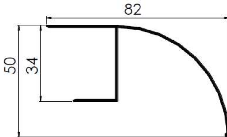
ARREMATE DIANTEIRO COMERCIAL (NOVO)
