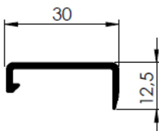
PERFIL LATERAL MESA 30 X 12,5 MM
