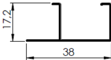
PUXADOR 38 X 17,2MM MV-15
