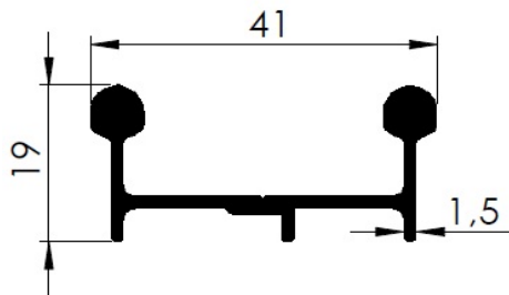
TRILHO DUPLO P/ CONJ. DESLIZANTE
