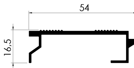
PROTETOR LATERAL BOIADEIRA
