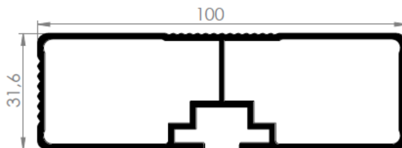
TRAVESSA LATERAL "NOVA"
