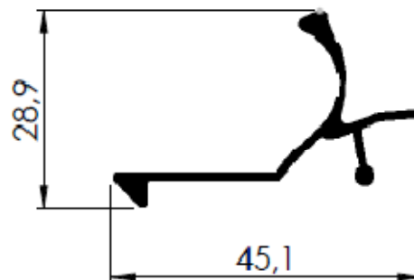
BATE FECHA (MOVEL 1570)
