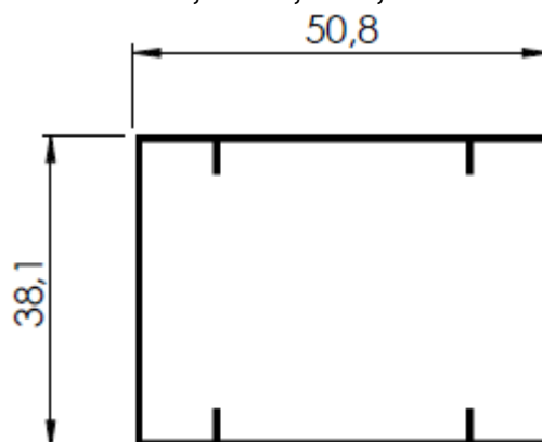
TUBO RETANGULAR (FRISO INTERNO) 50,8 X 38,1 X 0,95
